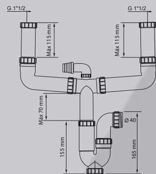
ESQUEMA DE COTAS
