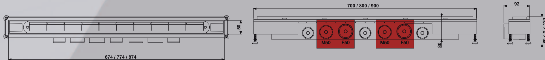
ESQUEMA DE COTAS
